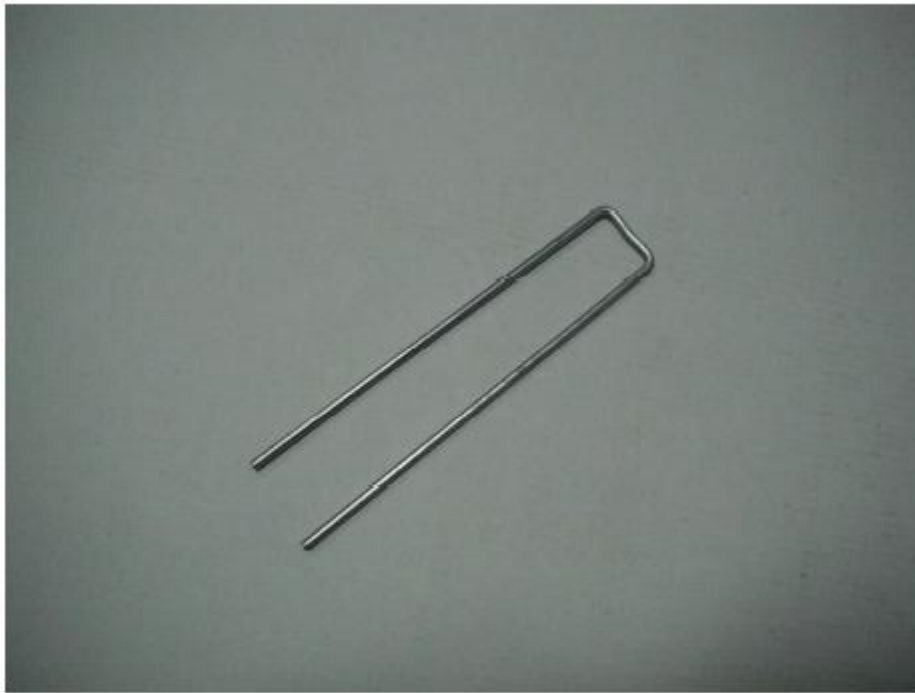
GC3/1515 - Grapa alambre galvanizada, Ø 3 mm., base 29, - altura 150 x 150 mm. En bolsas de 25 unidades.
