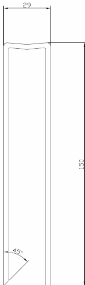
GC3/1515 - Grapa alambre galvanizada, Ø 3 mm., base 29, - altura 150 x 150 mm. En bolsas de 25 unidades.
