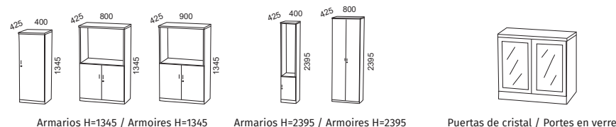
Armarios H=1345 / Armoires H=1345
