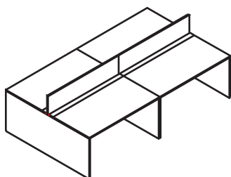
2xB20004= 2800*1650
