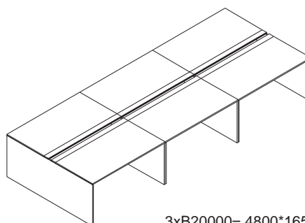
3xB20000= 4800*1650
