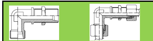
PASATABIQUES 90°
