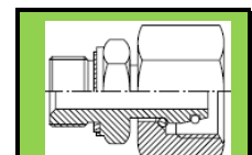
MACHO BSPP TUERCA LOCA DIN
