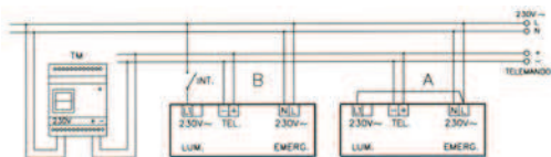
ESQUEMA DE CONEXIONES
